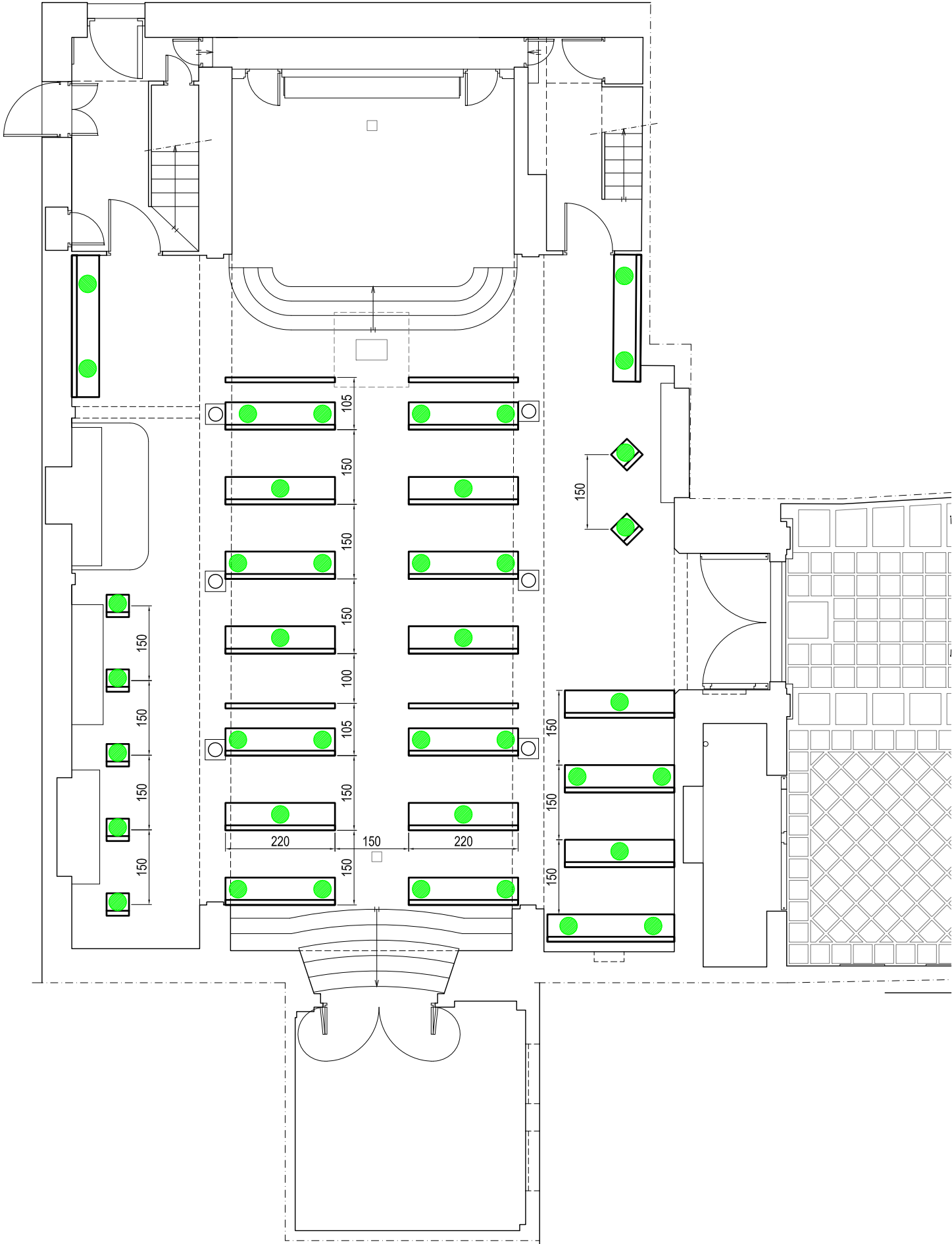
Sección horizontal a +1,50 m
